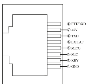
(Pin Belegung der Buchse)
