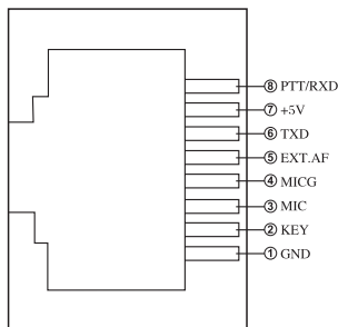
Spina del microfono (vista frontale)
