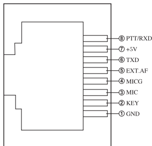
Mikrofonstecker (Draufsicht von vorne)
