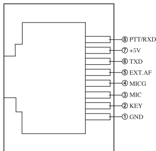
Prise microphone (vue de face)
